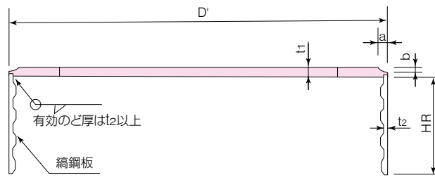
【R型（縞鋼板式）】 (全長PRC杭、PHC杭B種以上の性能の杭と継ぐ場合)
