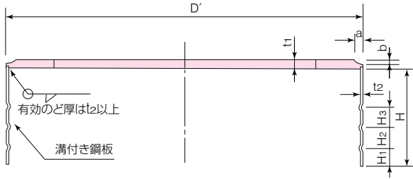
TYPE I (A種の杭、A種と継ぐ杭)
