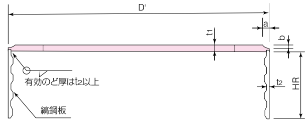
【R型(溝鋼板式)】
