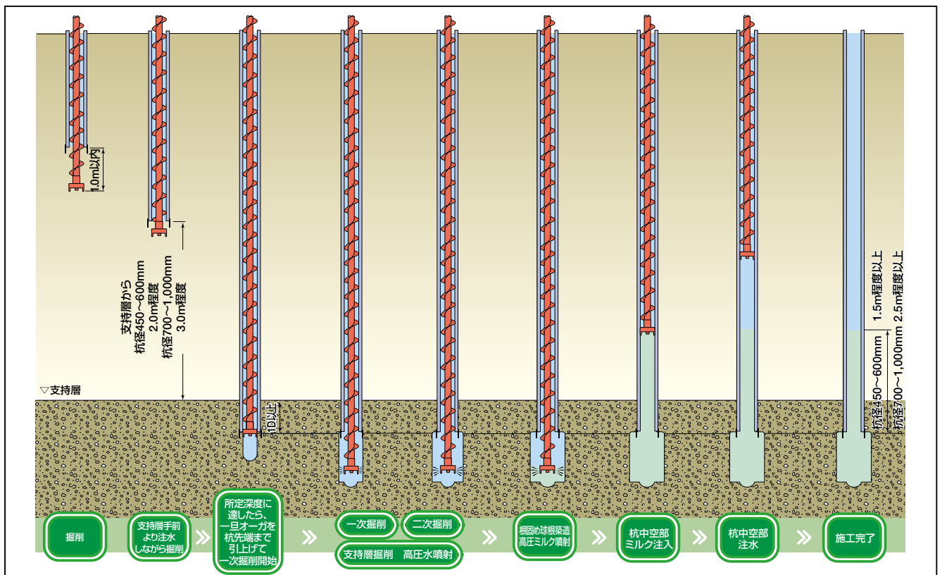
STJビット高圧噴射地上試験
