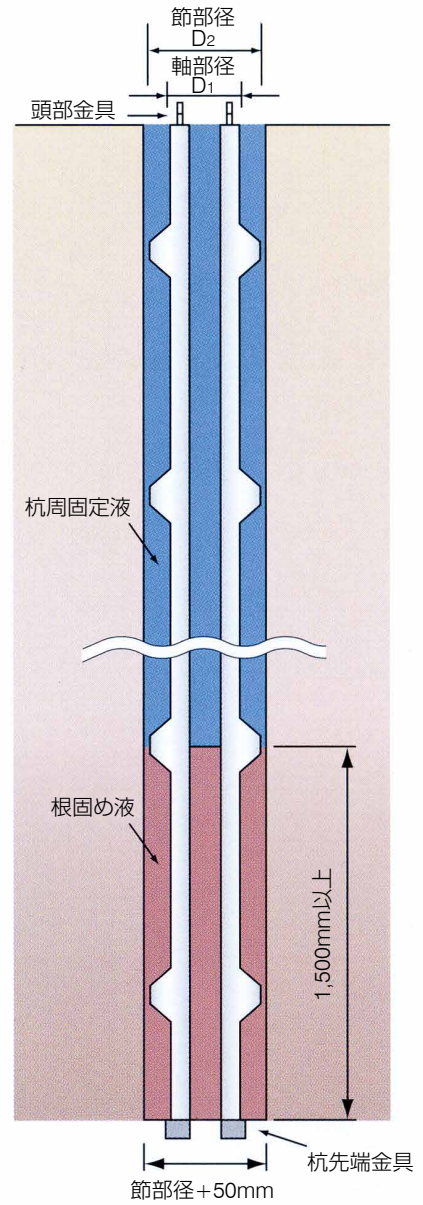
【杭施工完成図】
