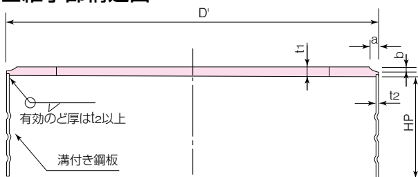
【P型】 (部分PRC杭で、PHC杭A種と継ぐ杭)
