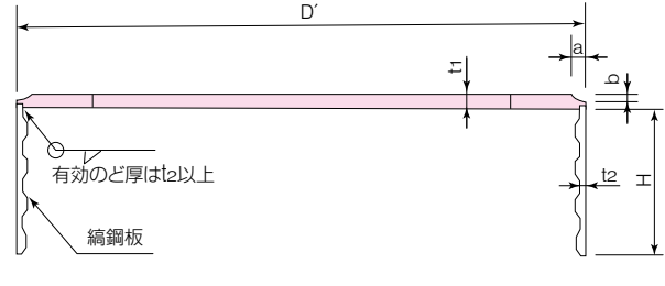
TYPE II (B種以上の性能を持つ杭同士を継ぐ場合)
