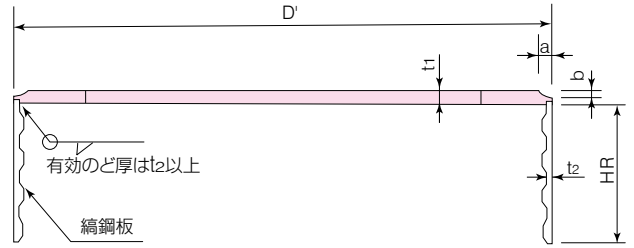
【R型(溝鋼板式)】
