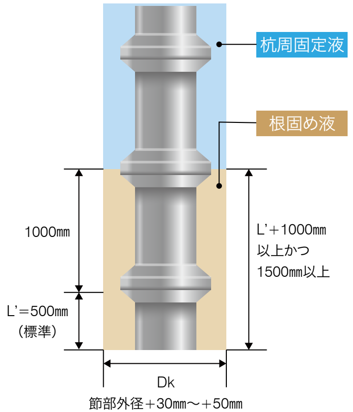
【根固め球根築造図】
