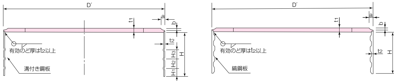
TYPE I (A種の杭、A種と継ぐ杭)
